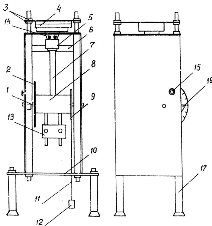
Схема стенда "ПРЯМОЙ УДАР":
