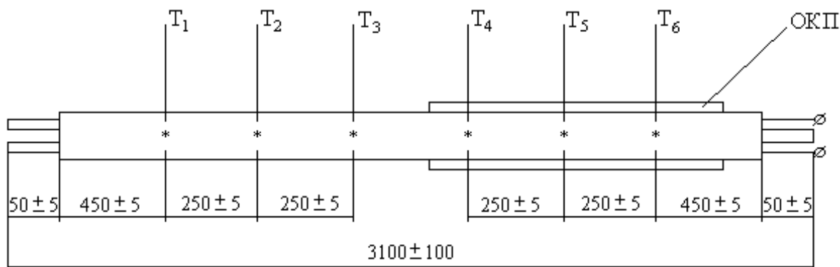
Размещение термоэлектрических преобразователей
