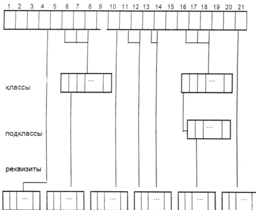
Рис.2. Структура классификатора
